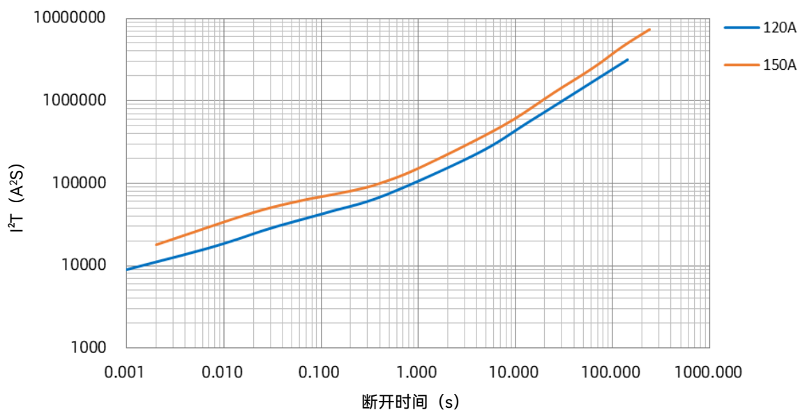
SKT-P I²t-t 曲线
